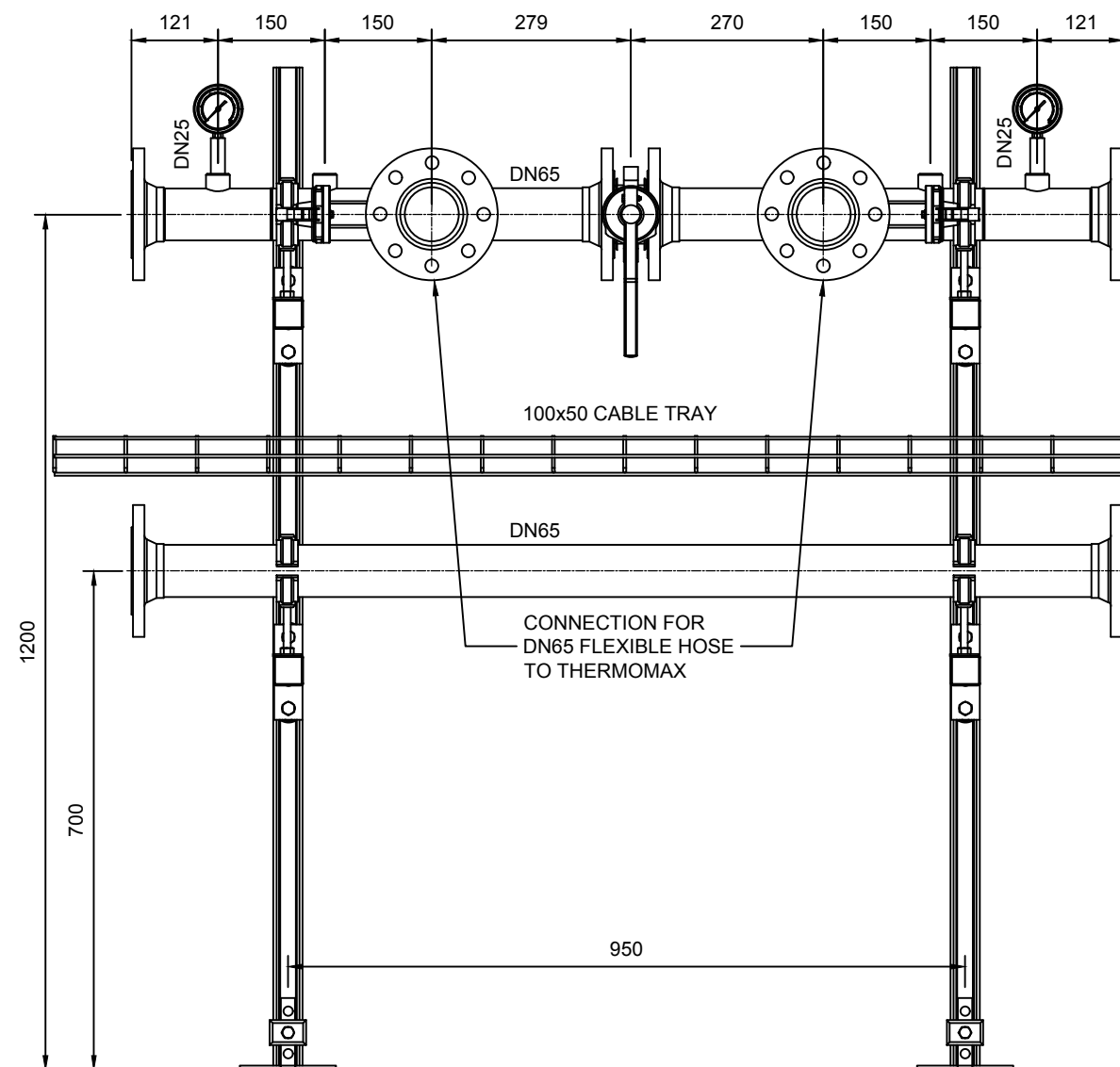
ELEVATION
